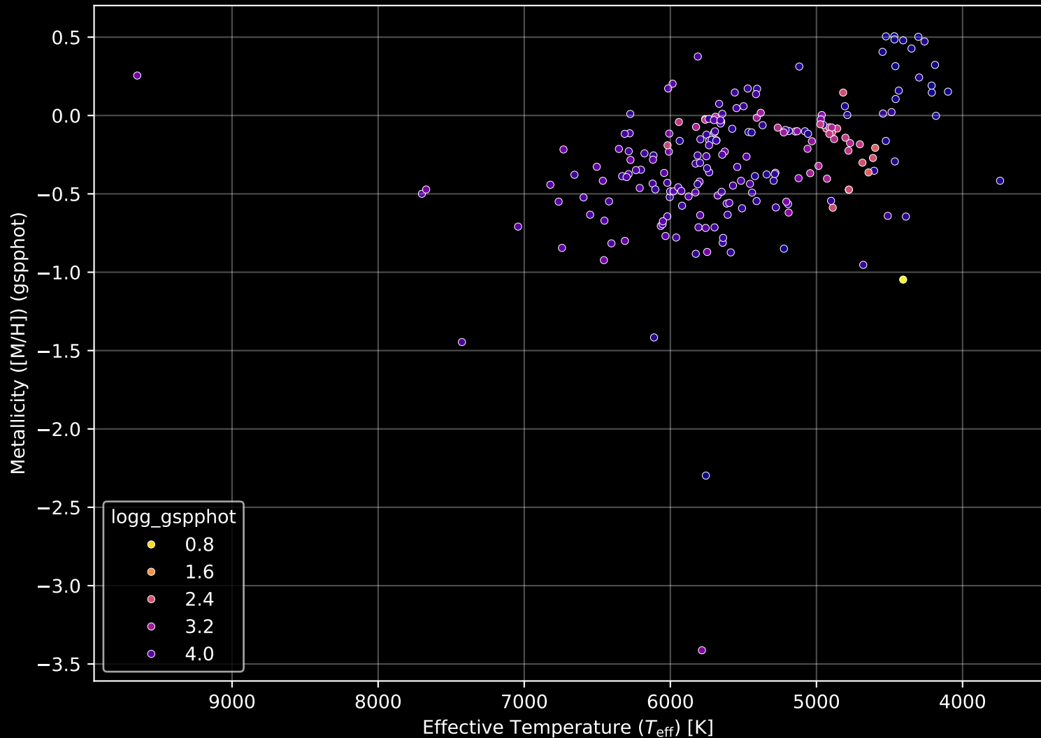
APOGEE DR17 Field: [K2_C12_082-57_btx] Stellar Population Parameters (n= 205)
